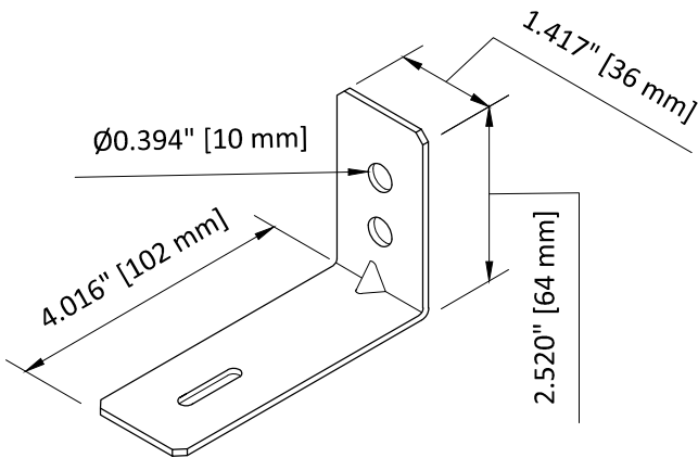
TUBRISE SQUARE BRACKET
